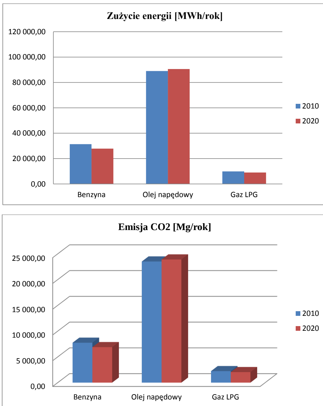
Rysunek 17. Zużycie energii i emisja CO 2 w transporcie w 2010 wraz z prognozą na rok 2020
