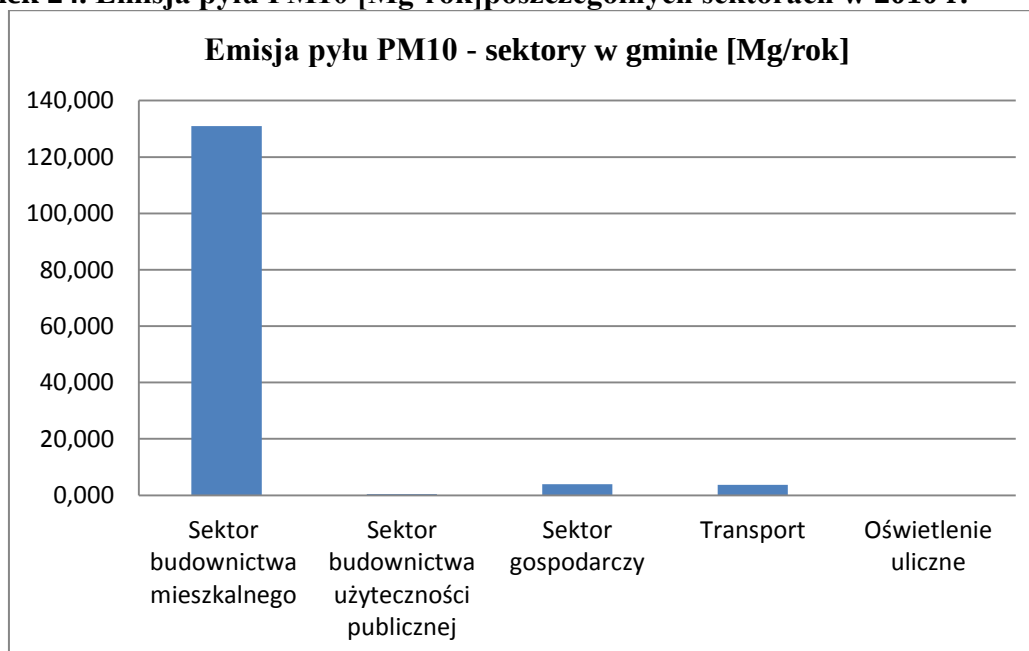
Rysunek 24. Emisja pyłu PM 10 [Mg-rok]poszczególnych sektorach w 2010 r.
