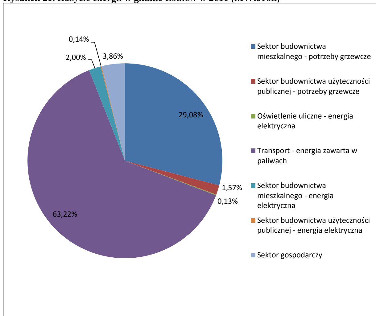
Rysunek 20. Zużycie energii w gminie Łonów w 2010 [MWh/rok]
