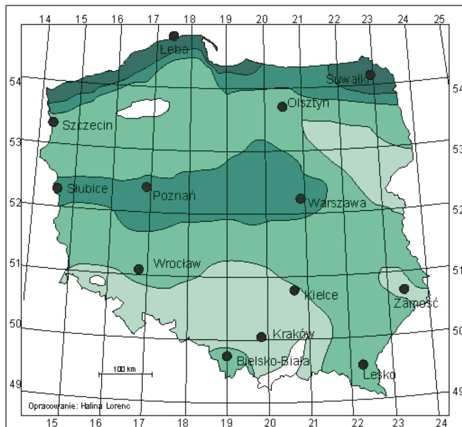
Rysunek 27. Strefy energetyczne wiatru w Polsce .
