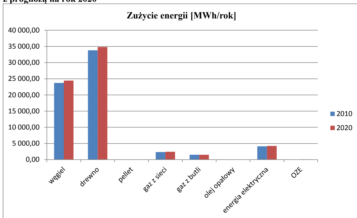
Rysunek 13. Zużycie energii i emisja CO 2 w budynkach mieszkalnych w 2010 wraz z prognozą na rok 2020
